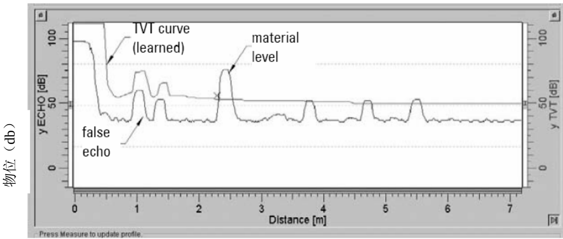
距离 (米)
