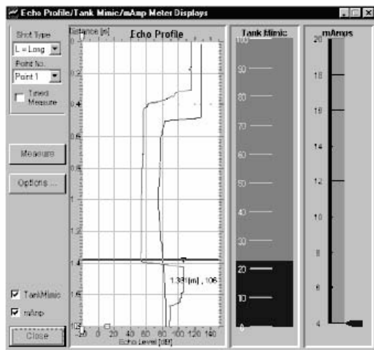
显示回波
